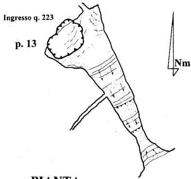
PIANTA
